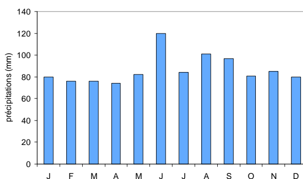
Figure 6 : Précipitations moyennes à Contamine sur Arve pour l'année 1999 ( www.meteofrance.fr )
