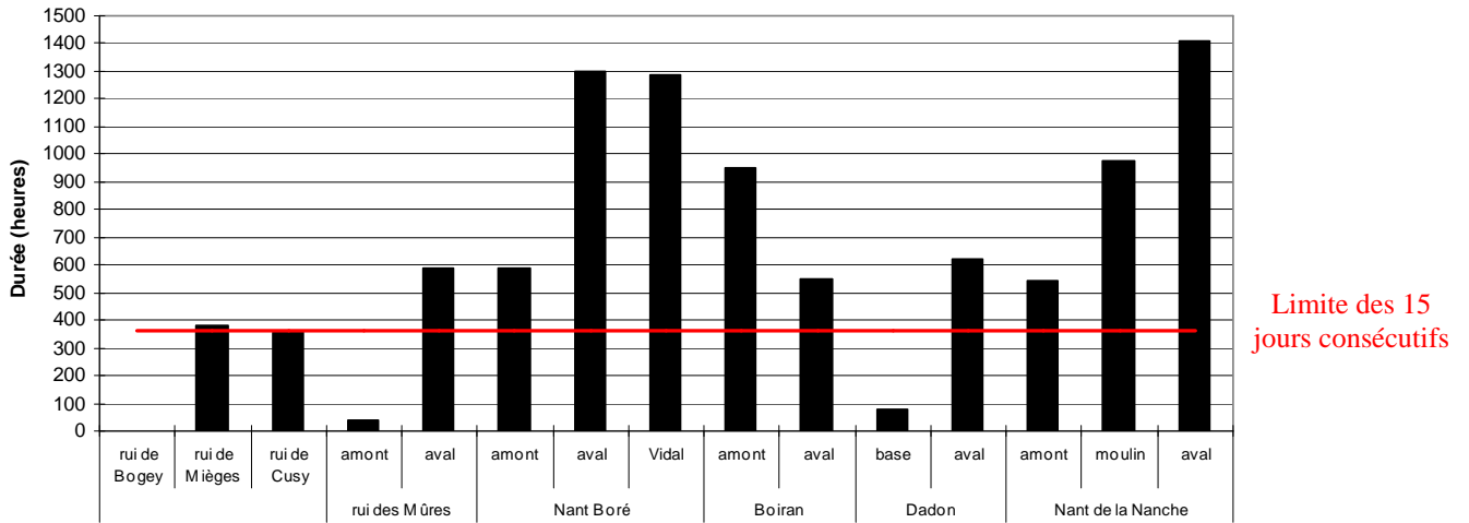
Figure 10: Durée en heures de la séquence maximale durant laquelle la température est restée au dessus de 15°C sur les 15 stations concernées par le suivi thermique réalisé sur les années 2005-2006 sur le bassin du Chéran.
