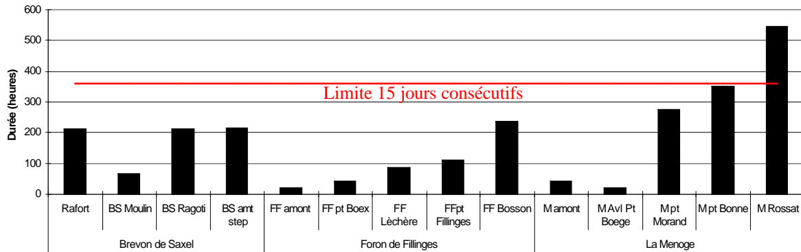
Figure 8 : Durée en heures de la séquence maximale durant laquelle la température est restée au dessus de 15°C sur les 14 stations concernées par le suivi annuel sur la Menoge et ses affluents.
