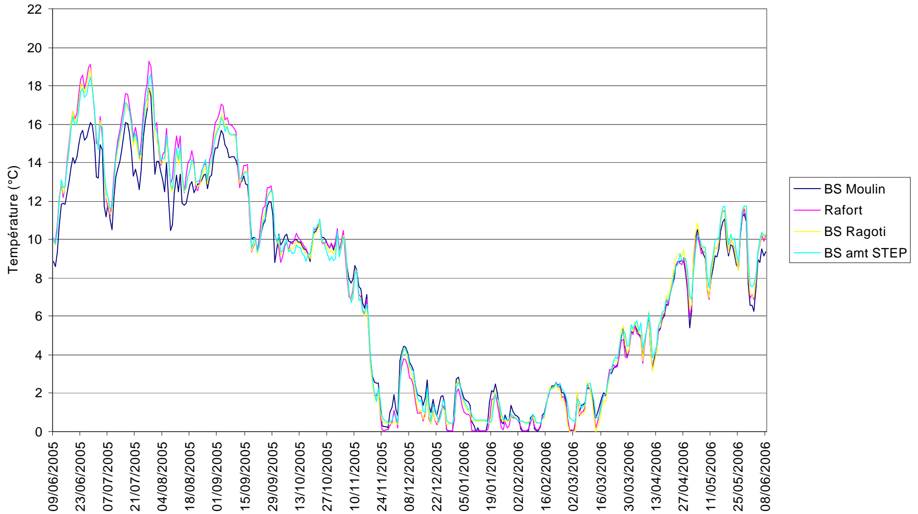
Figure 4 : Courbes des températures moyennes journalières calculées sur la période du 09/06/2005 au 08/06/2006 pour les 4 stations étudiées sur le Brevon de Saxel, affluent de la Menoge.
