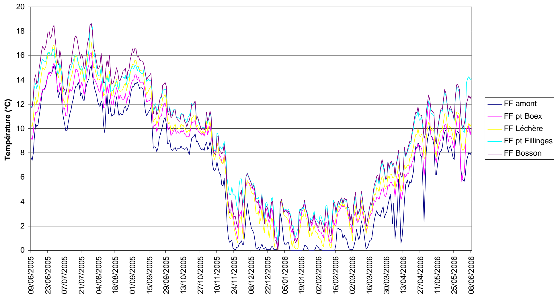
Figure 5 : Courbes des températures moyennes journalières calculées sur la période du 09/06/2005 au 08/06/2006 pour les 4 stations étudiées sur le Foron de Fillings, affluent de la Menoge.
