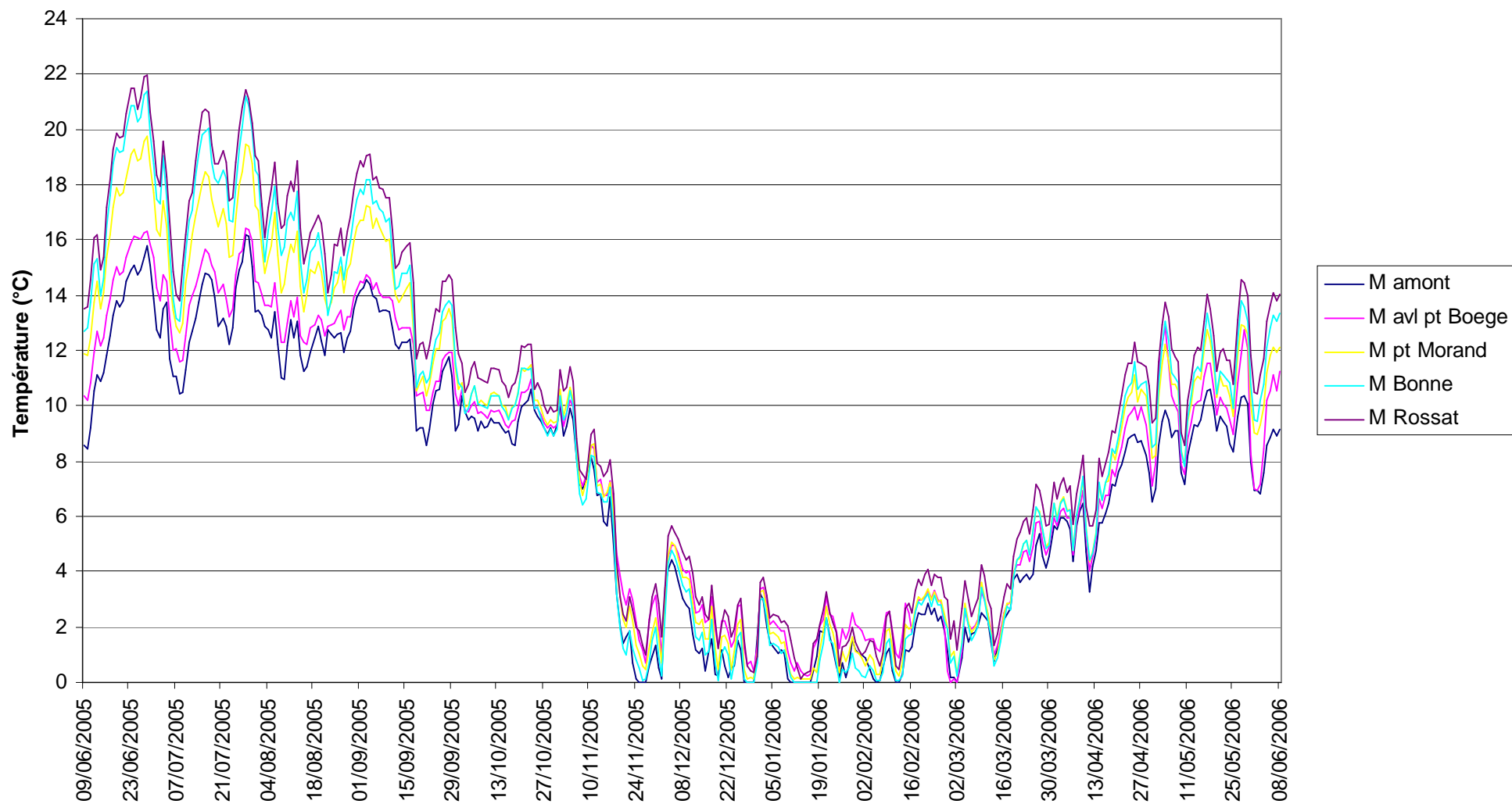
Figure 3 : Courbes des températures moyennes journalières calculées sur la période du 09/06/2005 au 08/06/2006 pour les 5 stations étudiées sur le cours principal de la Menoge.
