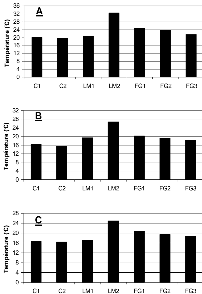
Figure 3 : Température maximale (A), amplitude journalière moyenne annuelle (B) et moyenne des trente jours les plus chauds (C) obtenues sur les 6 stations concernées par le suivi thermique annuel sur le Foron.
