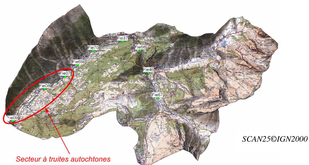
Figure 5 : Répartition des truites autochtones sur le bassin versant du Nom (Caudron, 2008)
